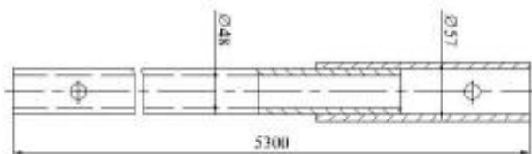
Анкер крепления
