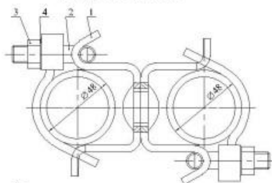
Хомут поворотный
