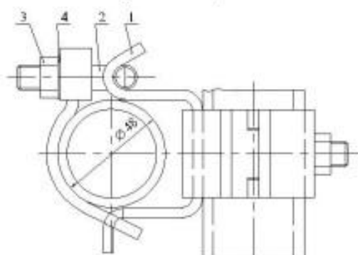
Хомут поворотный
